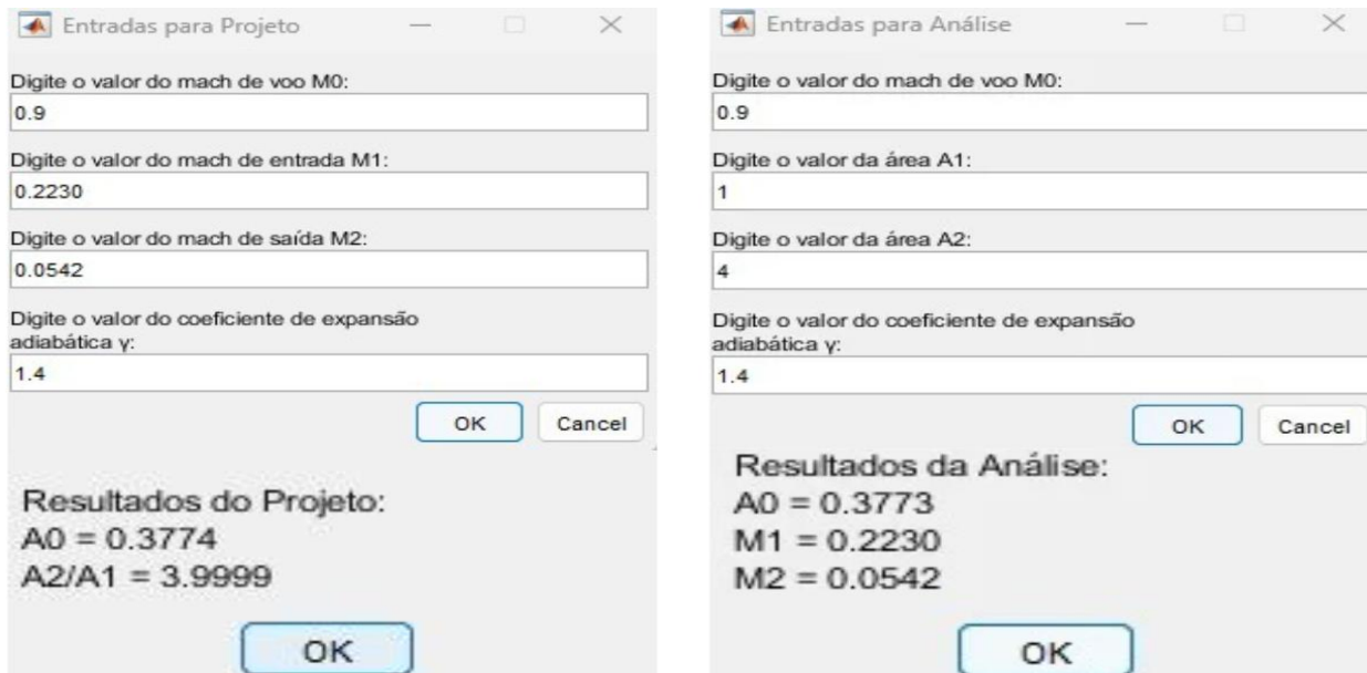
FIGURA 1. Interfaces de resultados do projeto para Machs especificados (à esquerda) e de análise para áreas especificadas (à direita).
