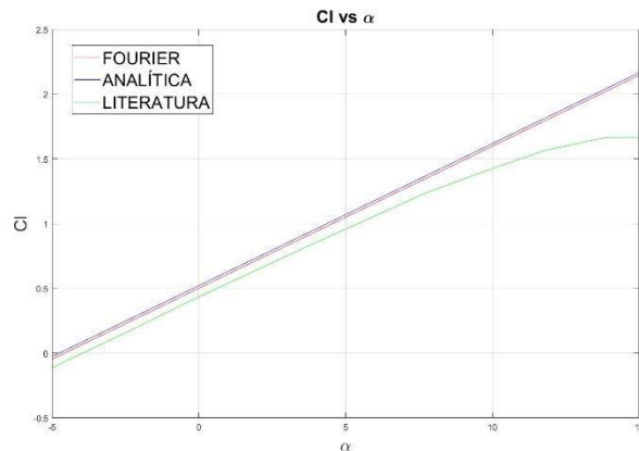
Figura 2: coeficiente de sustentação
