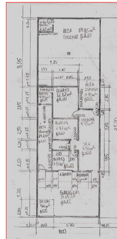
PLANTA BAIXA À MÃO
